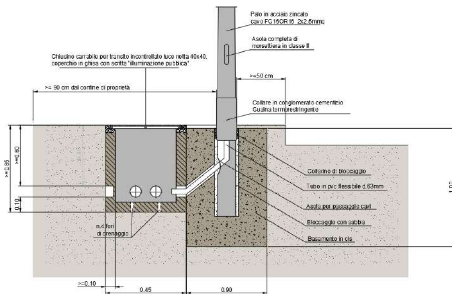
Figura 1 Plinto di fondazione per pali di altezza fuori terra fino a 5.00 metri
