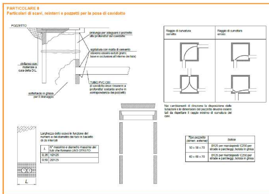
Figura 3 – Scavi, reinterri e pozzetti per la realizzazione di cavidotti
