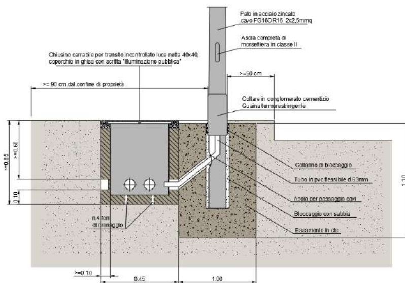
Figura 2 Plinto di fondazione per pali di altezza fuori terra oltre i 5.00 metri
